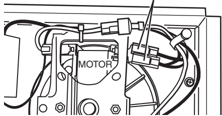
FIG. 10 - 120VAC TO 240VAC CONVERSION CONVERSIÓN DE 120VCA A 240VCA
